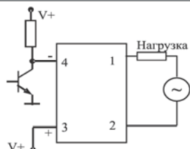
NPN, нормально-разомкнутый
