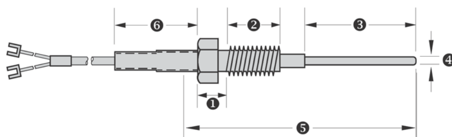
Датчик типа TS-2
