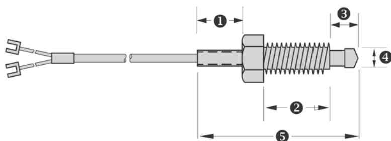
Датчик типа TS-2
