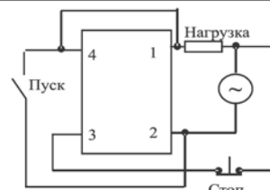
Схема с самоблокировкой (АС-АС)
