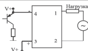
PNP, нормально-замкнутый
